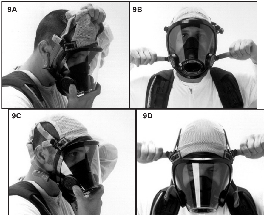
FIGURA 9 COLOCACIÓN DE LA PIEZA FACIAL DE CUATRO CORREAS
